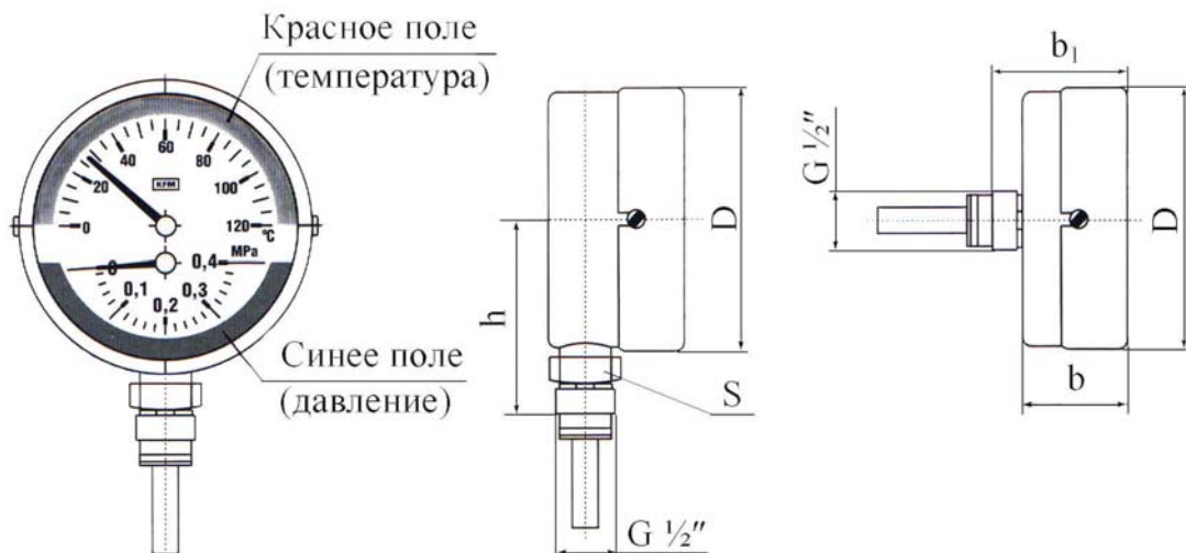
Радиальное присоединение
