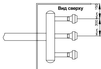
Рис 4 Варианты монтажа двух и трех инжекторов
