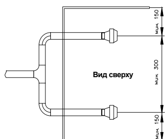
Рис 4 Варианты монтажа двух и трех инжекторов
