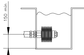
Рис 5 монтаж одиночного инжектора
