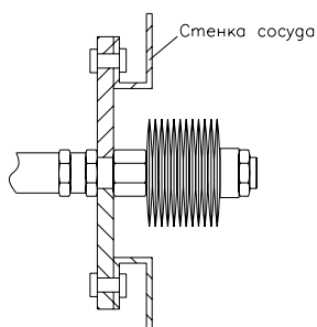
Рис 3 Монтаж на плите с приборной рамой
